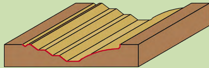
№ 11 Сечение фасада – «Палеро»
