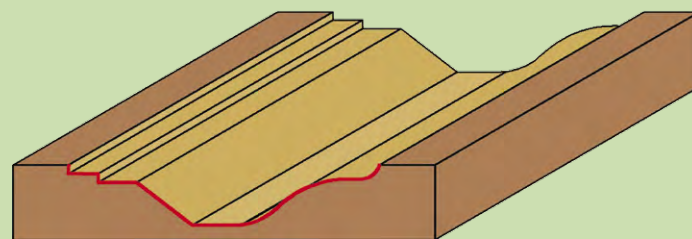
№ 12 Сечение фасада – «Сорренто»
